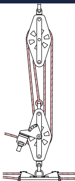
6:1 MAINSHEET
