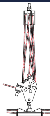
6:1 MAINSHEET PLUS 24:1 FINE TUNE
